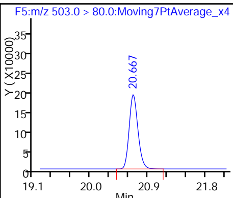
* 8 13C4 PFOS
