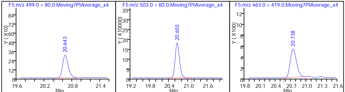
$ 10 13C2 PFDA
