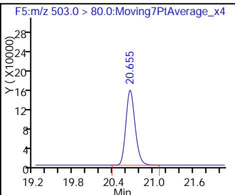
* 8 13C4 PFOS
